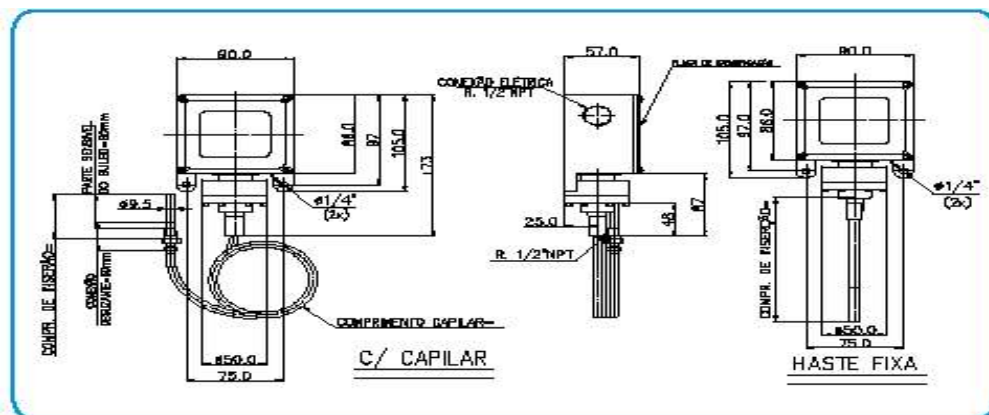
DESENHO DIMENSIONAL
