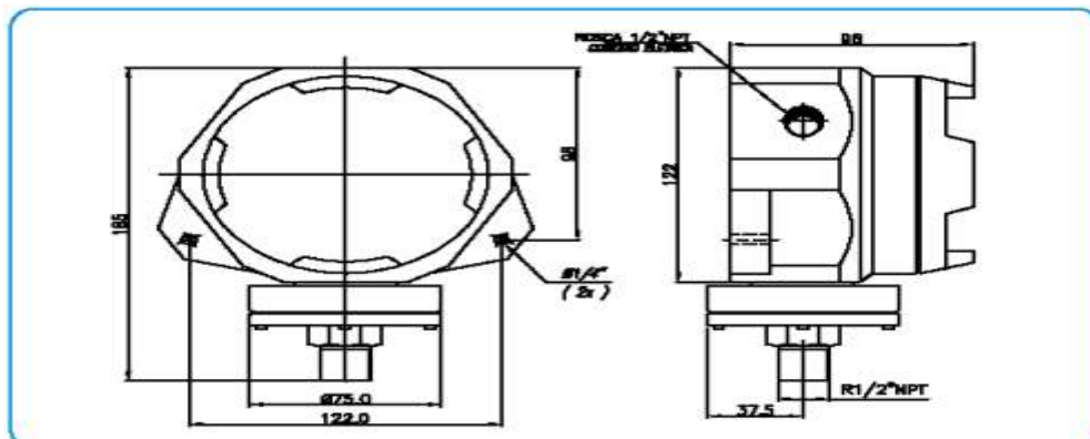
DESENHO DIMENSIONAL
