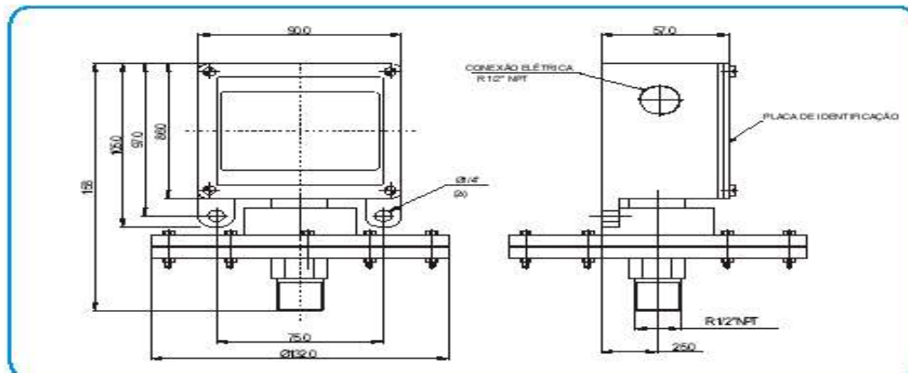
DESENHO DIMENSIONAL Série WPBP-7000
